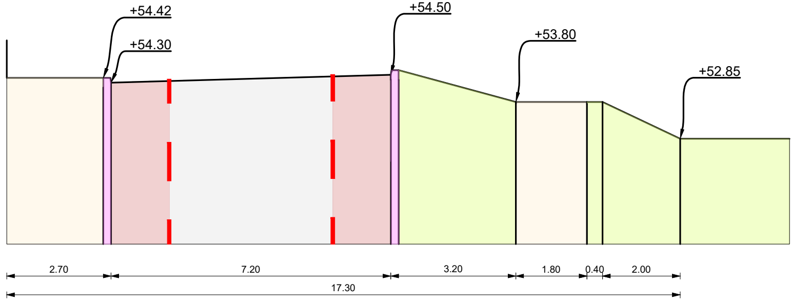
Dwarsprofiel A - A bestaande situatie Schaal 1:100
