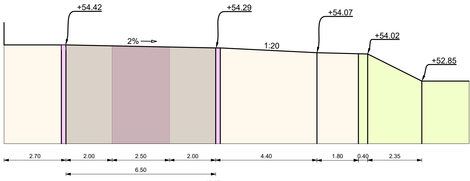
Dwarsprofiel A - A nieuwe situatie Schaal 1:100
